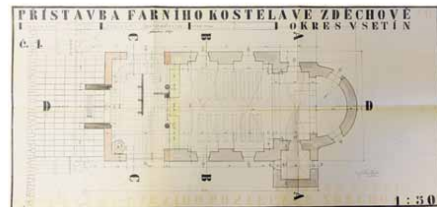
Plán přístavby kostela z roku 1941
